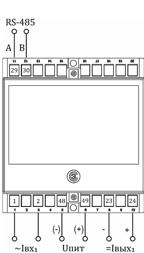
а) Корпуса E20 (1 вход, 1 аналоговый выход, 1 порт RS-485)
