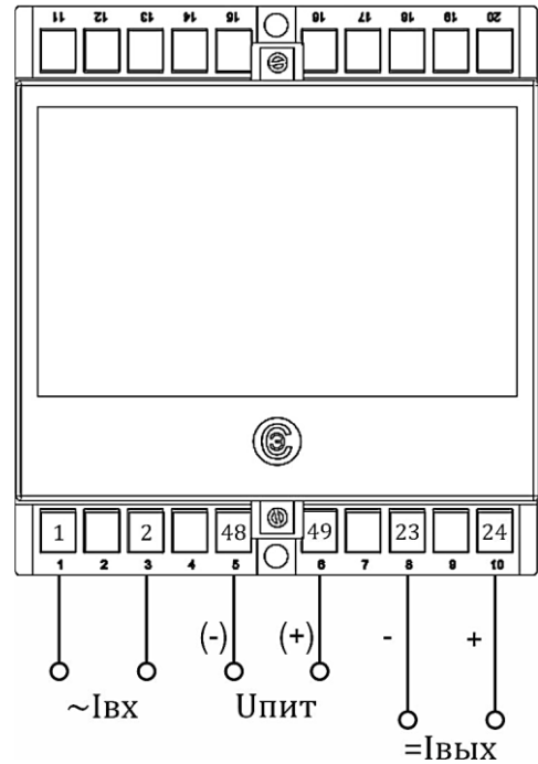
г) Копус Е20 (1 вход, 1 аналоговый выход)
