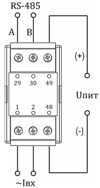
б) Копус М6 (1 вход, 1 порт RS-485)
