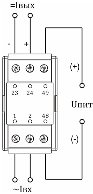
а) Копус М6 (1 вход, 1 аналоговый выход)
