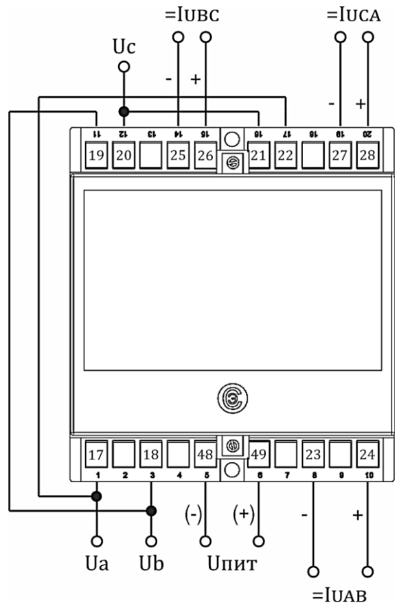
б) Корпус E20 (3 входа, 3 аналоговых выхода) схема для контроля междуфазных напряжений
