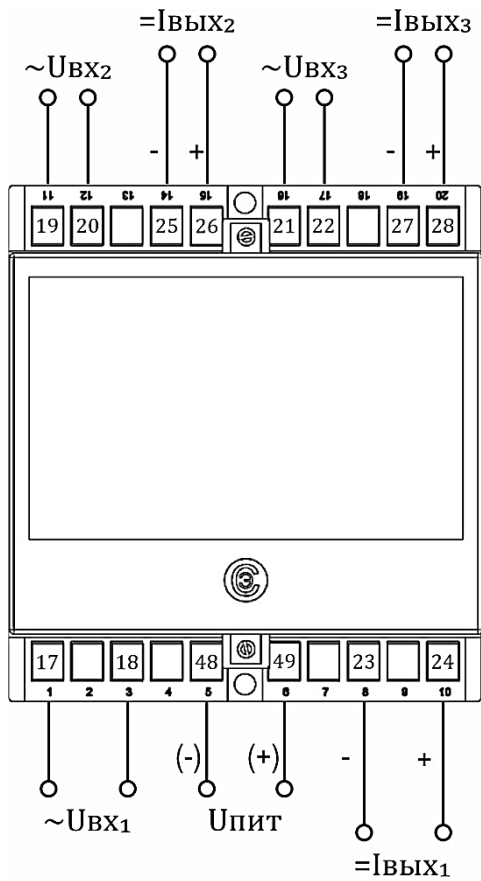
а) Корпус E20 (3 входа, 3 аналоговых выхода) схема для контроля фазных напряжений
