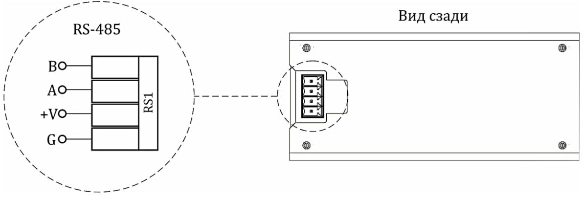
Рисунок Б.9 – Схемы электрические подключения E8DU
