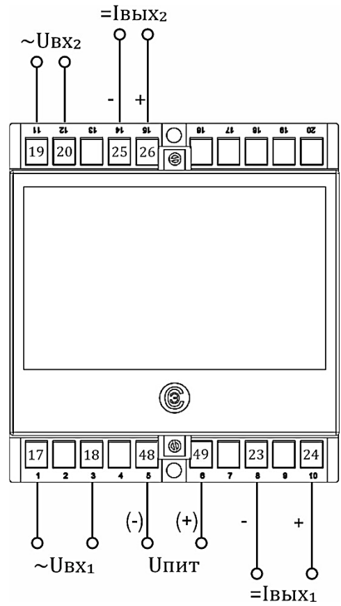
б) Корпус E20 (2 входа, 2 аналоговых выхода)
